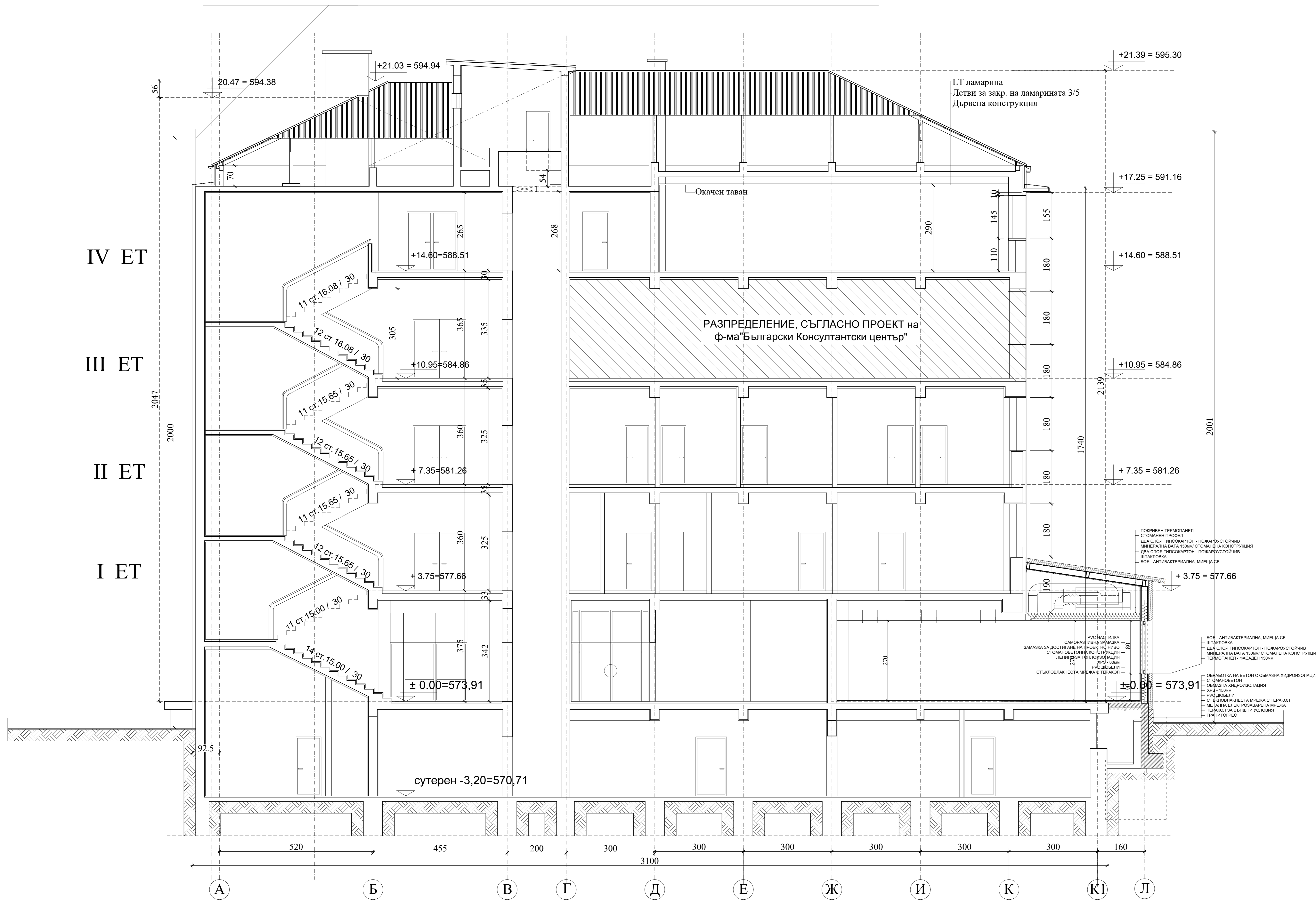
РАЗРЕЗ А-А М 1:50
